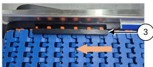
Abb. 4: Modulbandkette anpassen
