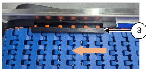
Abb. 3: Montage der Modulbandkette
